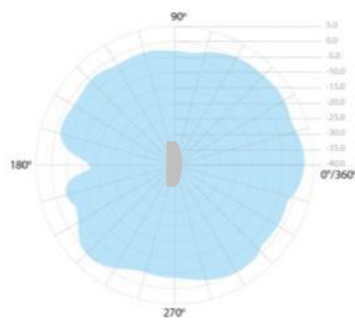
2.4GHz 2D Strahlungsdiagramm@ Vertikal
