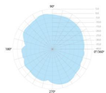
2.4GHz 2D Strahlungsdiagramm@ Horizontal
